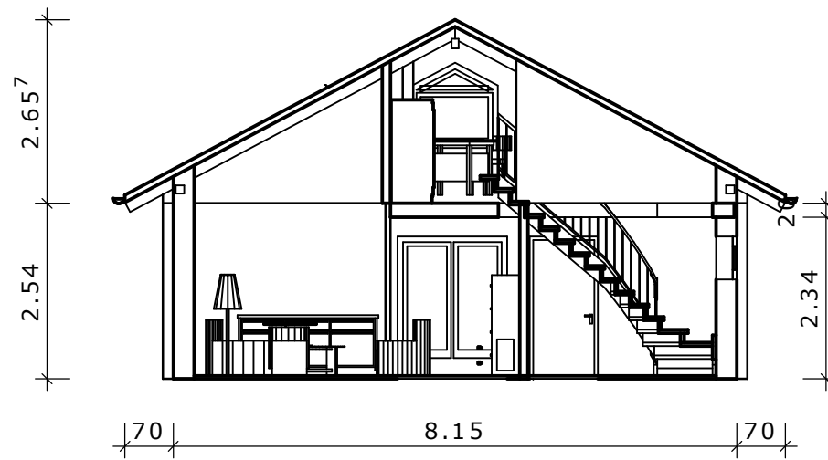
Schnitt a-a
